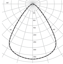
MODUL 02 02024-P2 DE 2666lm
